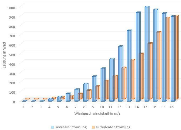
Leistungskennlinie SkyWind NG
